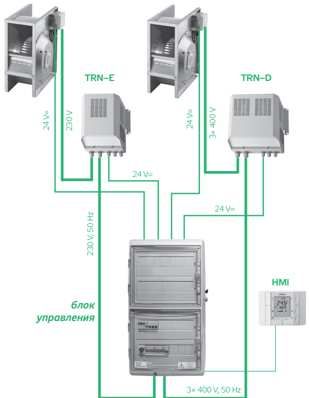
РИС. 8 – ПОДКЛЮЧЕНИЕ ВЕНТИЛЯТОРА
