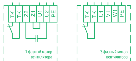
РИС. 6 – СХЕМЫ ПОДКЛЮЧЕНИЯ
