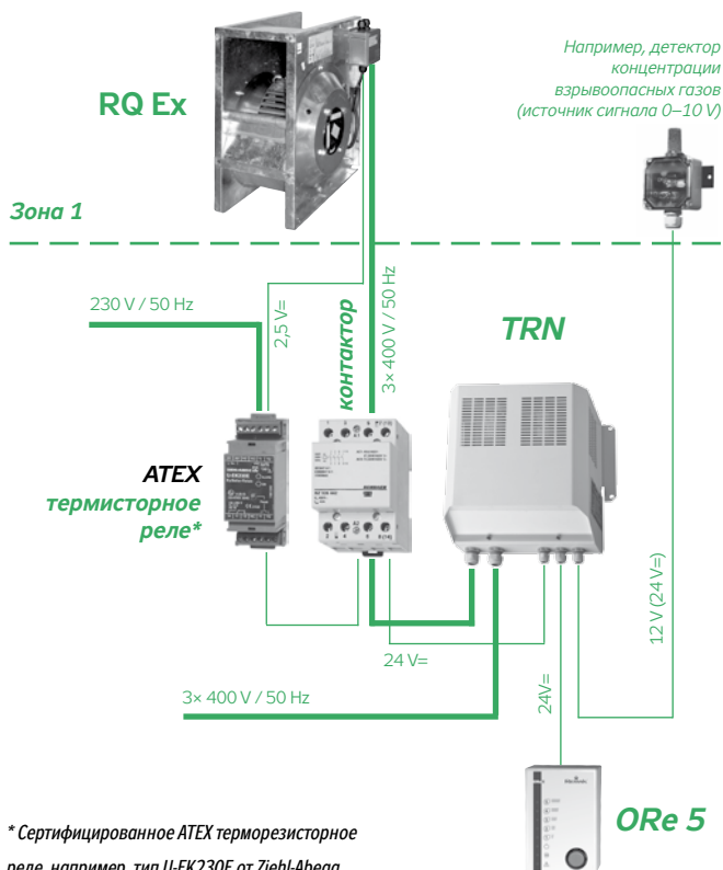
РИС. 12 – ПОДКЛЮЧЕНИЕ ВЕНТИЛЯТОРА
