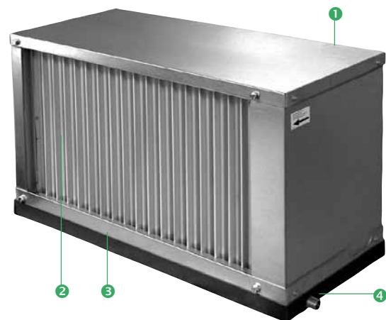
РИС. 3 – ОПИСАНИЕ ЧАСТЕЙ КАПЛЕУЛОВИТЕЛЯ
