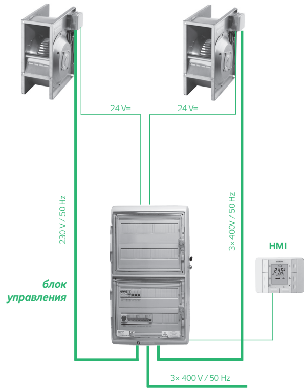
РИС. 7 – ПОДКЛЮЧЕНИЕ ВЕНТИЛЯТОРА
