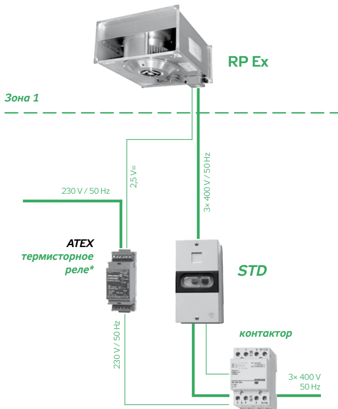
РИС. 11 – ПОДКЛЮЧЕНИЕ ВЕНТИЛЯТОРА
