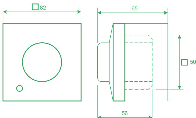
РИС. 46 – РАЗМЕРЫ РЕГУЛЯТОРА
