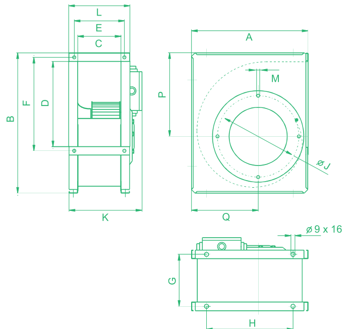
РИС. 2 – ОБОЗНАЧЕНИЕ РАЗМЕРОВ
