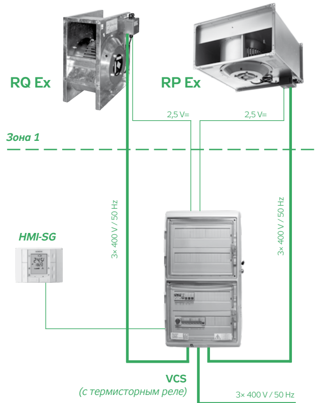
РИС. 13 – ПОДКЛЮЧЕНИЕ ВЕНТИЛЯТОРА
