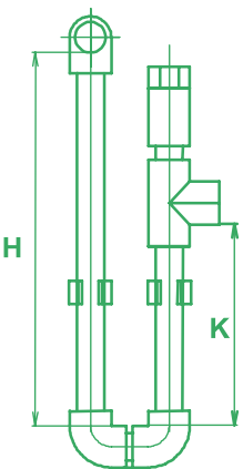
РИСУНОК 14 – ОТВОД КОНДЕНСАТА
