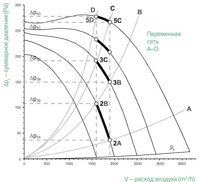
РИС. 3 – ХАРАКТЕРИСТИКА СЕТИ
