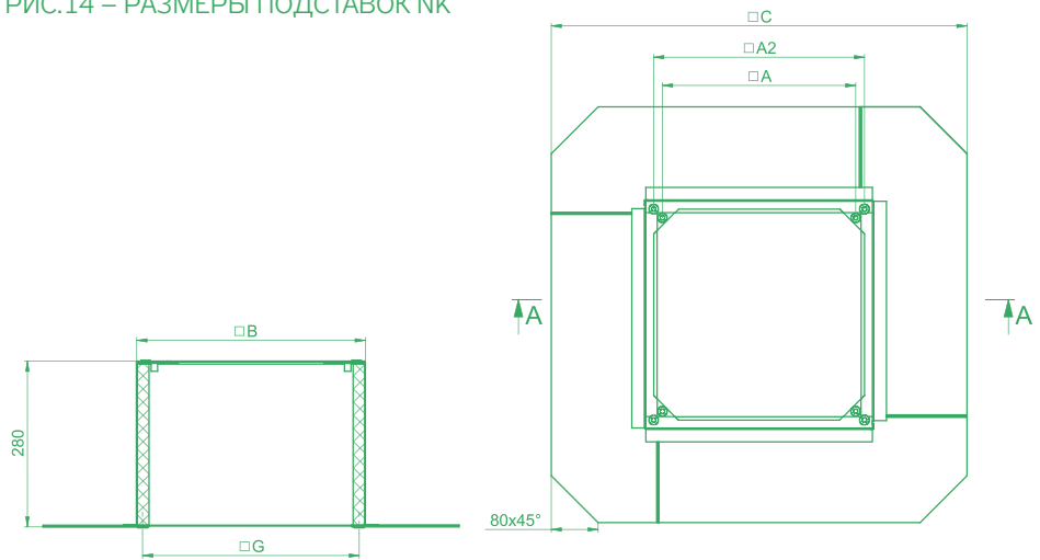
РИС.14 – РАЗМЕРЫ ПОДСТАВОК НК
